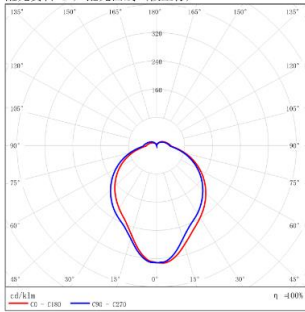
配光资料 1 / 配光曲线 (极坐标)
