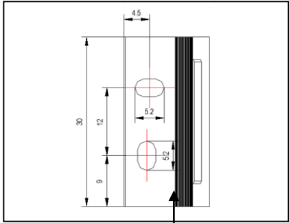
固定支架孔位尺寸
